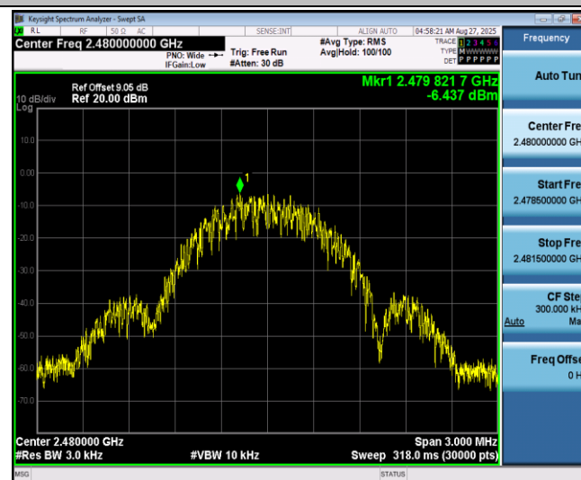
BLE_Ant1_2480
