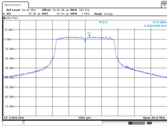
MIMO Ant. 1
