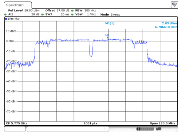
MIMO Ant. 2
