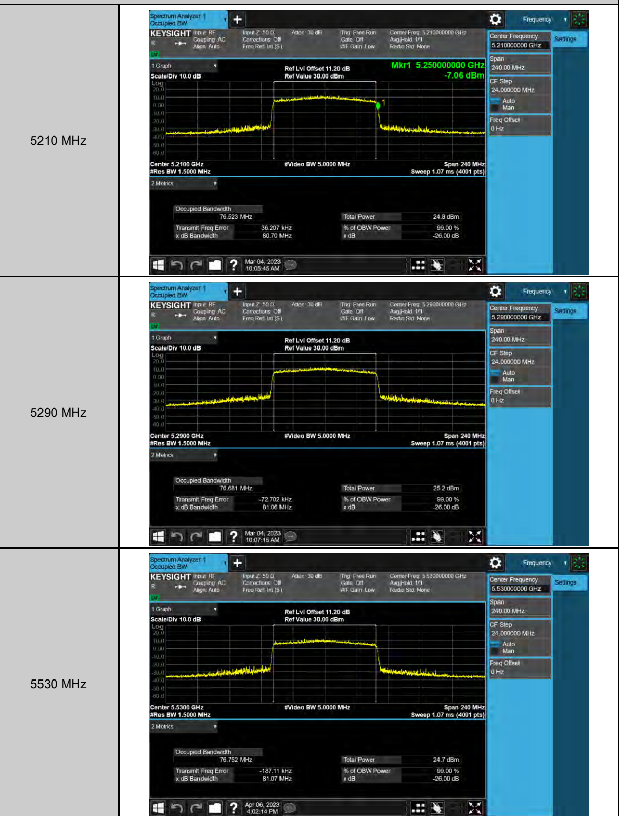
802.11ax HE80_ANT-3
