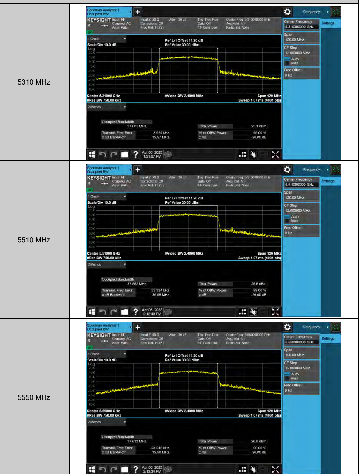
802.11ax HE40_ANT-3
