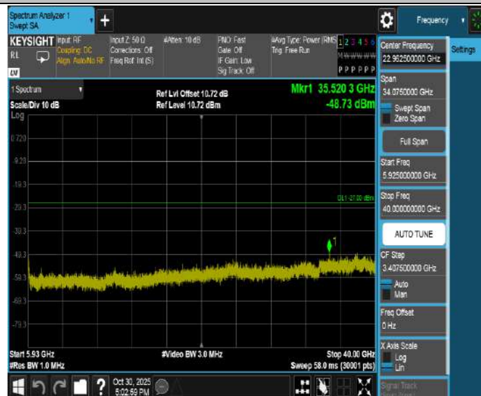
11AX20MIMO_Ant1_5180_30~5140
