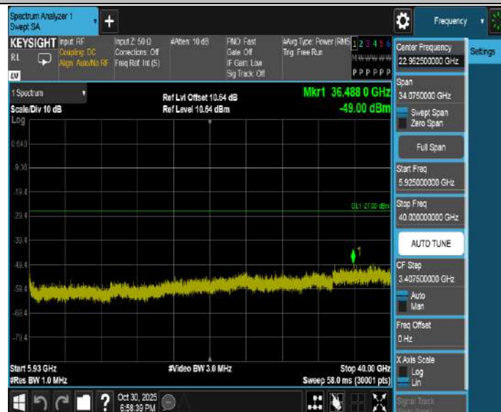
11AX20MIMO_Ant2_5825_30~5650
