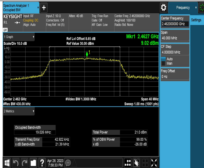
11AX20ISO_Ant2_2462
