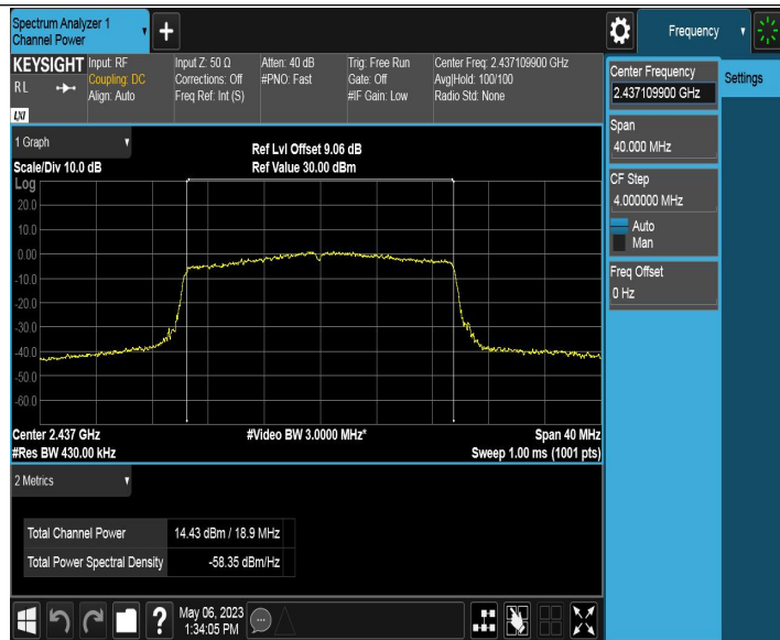
11AX20MIMO_Ant2_2437
