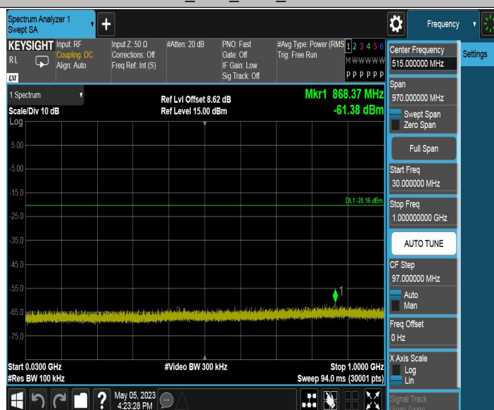
11G_Ant2_2462_30~1000
