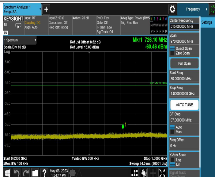
11AX20MIMO_Ant2_2437_30~1000
