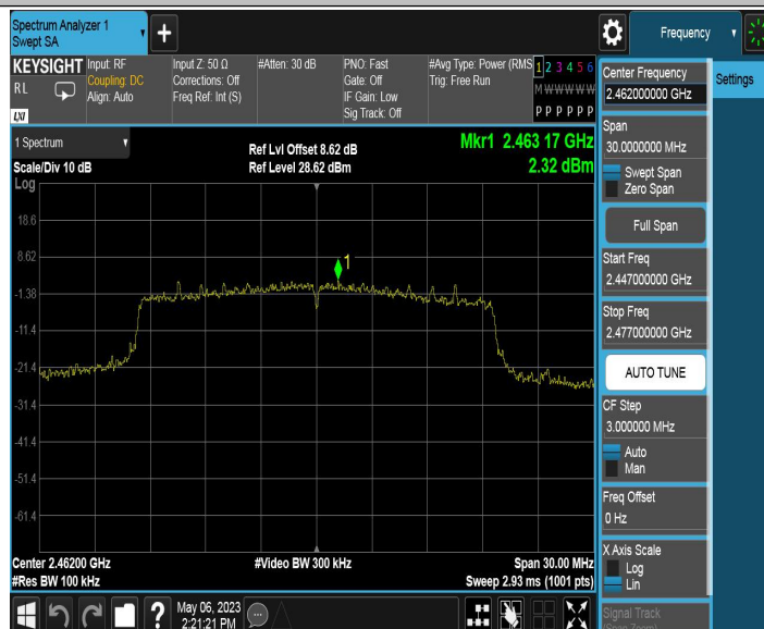
11AX20MIMO_Ant2_2462_0~Reference
