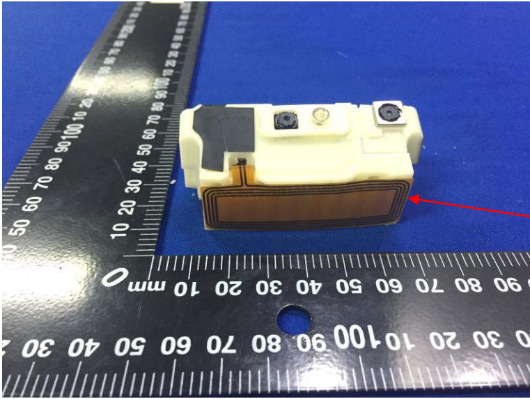
RFID Antenna
