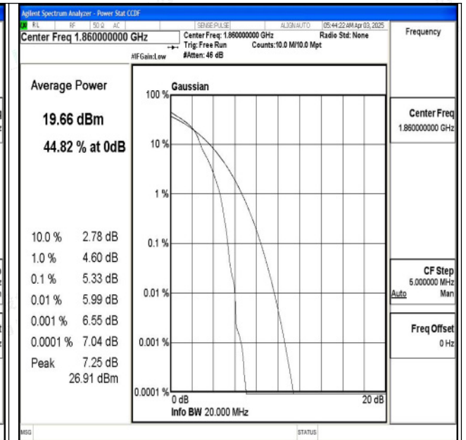
Band2-20MHz-16QAM-18700-1RB#0-PASS
