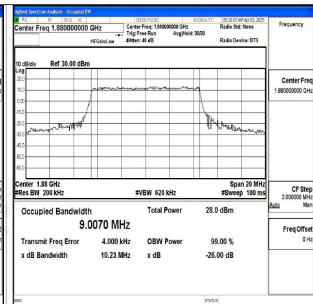
Band2-10MHz-16QAM-18900-50RB#0-PASS
