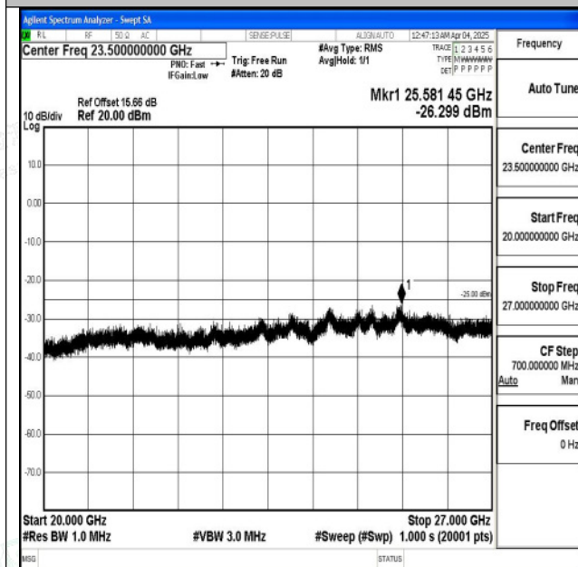
Band7_15MHz_QPSK_21100_1RB#0_20000~27000_20000~27000 000~27000
