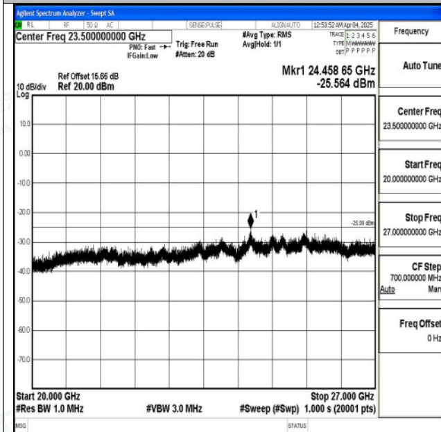
Band7_20MHz_QPSK_21350_1RB#0_20000~27000_20000~27000 000~27000
