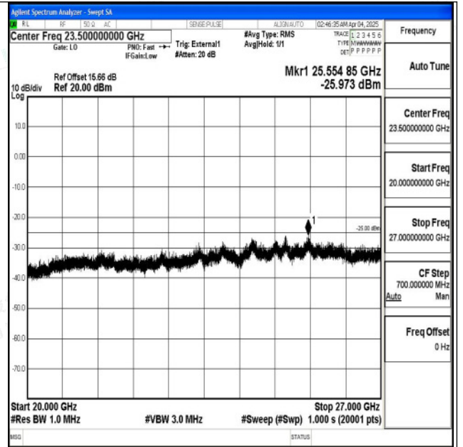
Band38_15MHz_16QAM_38175_1RB#0_20000~27000_2 20000~27000
