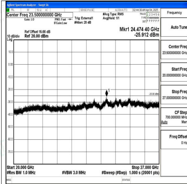
Band38_15MHz_QPSK_38175_1RB#0_20000~27000_2 0000~27000
