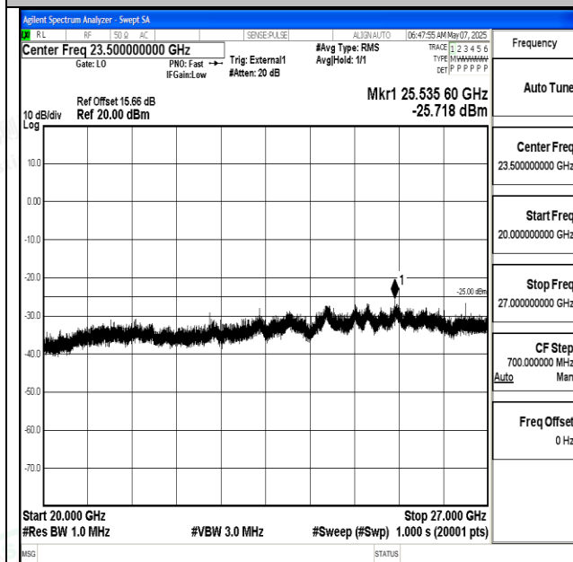
Band38_15MHz_QPSK_38000_1RB#0_20000~27000_2 0000~27000
