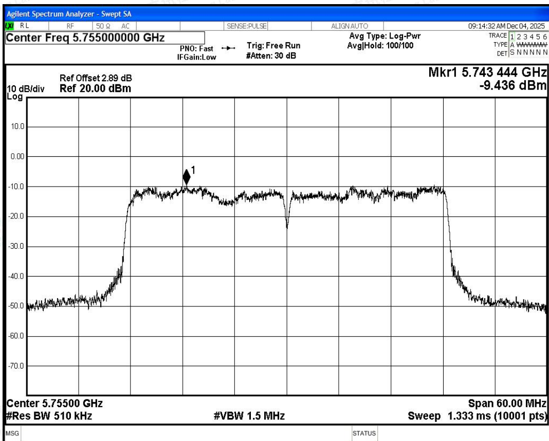
PSD NVNT ac40 5755MHz Ant1
