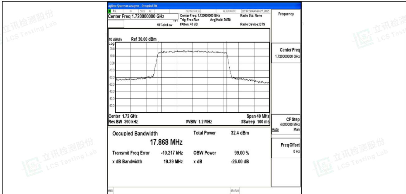
Band4-20MHz-QPSK-20050-100RB#0-PASS
