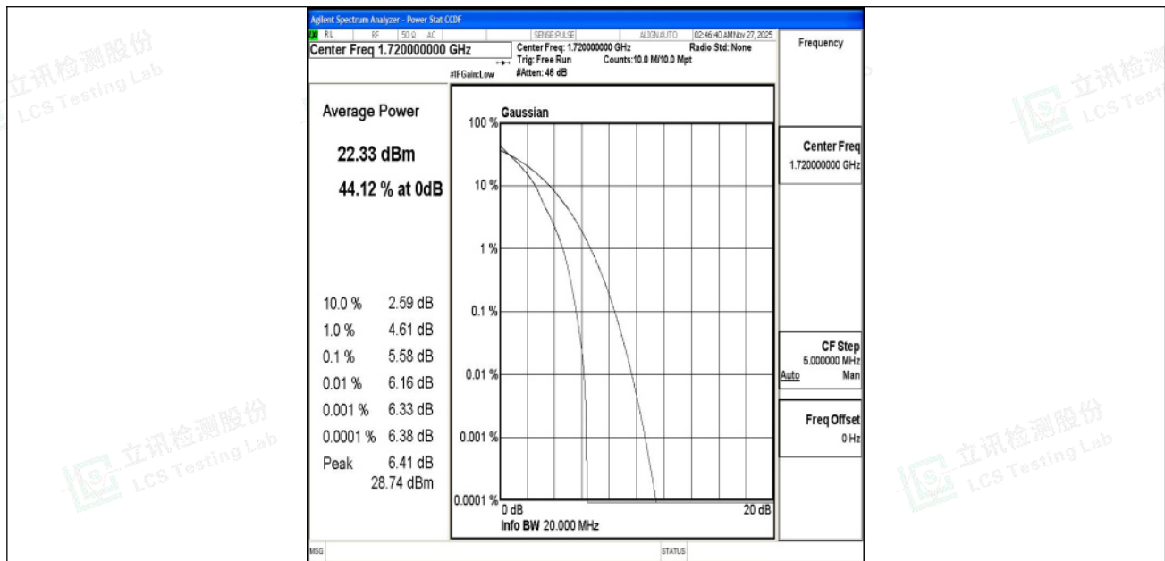
Band4-20MHz-QPSK-20050-1RB#0-PASS
