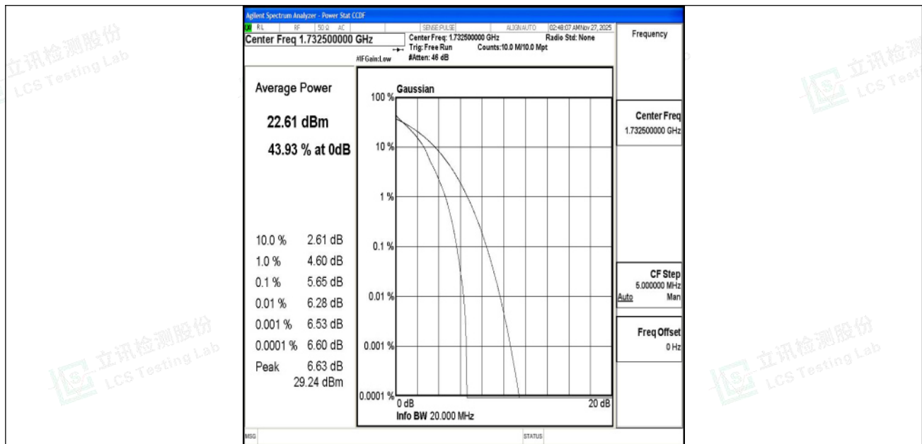
Band4-20MHz-QPSK-20175-1RB#0-PASS
