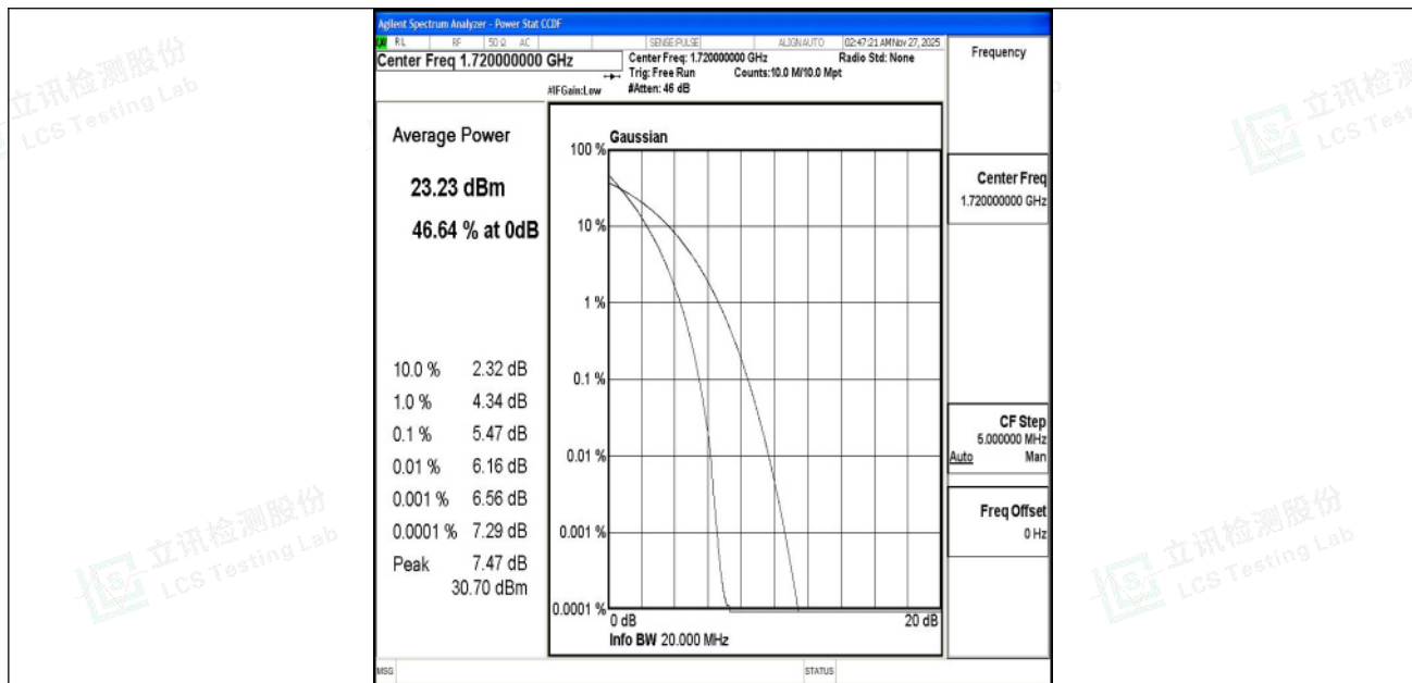
Band4-20MHz-QPSK-20050-100RB#0-PASS
