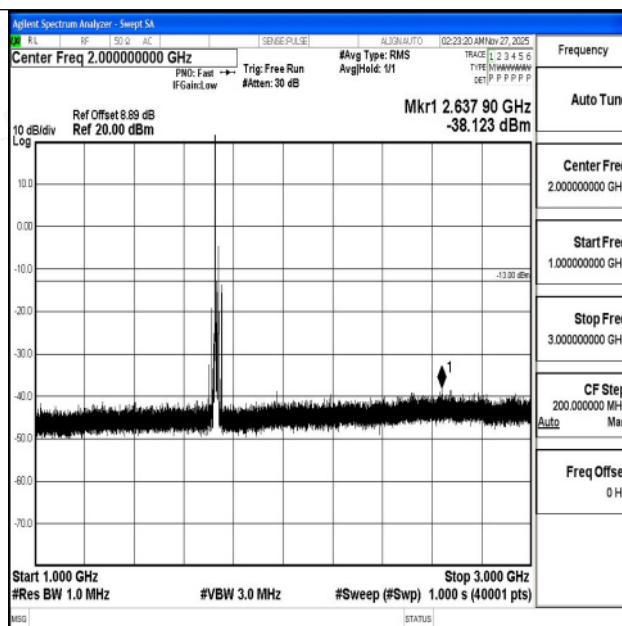
Band4 15MHz QPSK 20175 1RB#0 1000~3000 1000~3000
