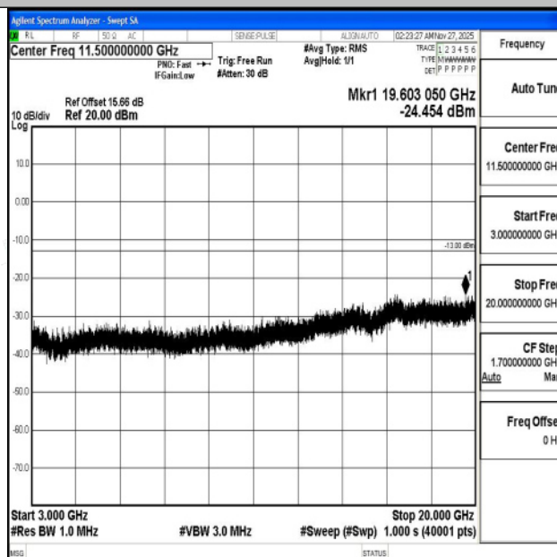
Band4 15MHz QPSK 20175 1RB#0 3000~20000 3000~20000
