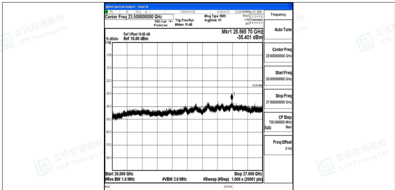
Band7_20MHz_QPSK_20850_1RB#0_20000~27000_20000~27000
