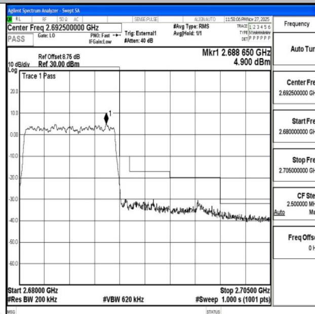
Band41_10MHz_QPSK_41540_50RB#0
