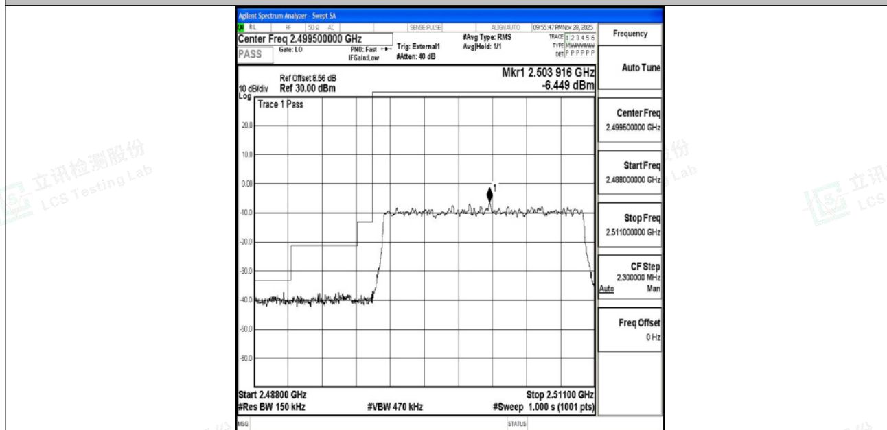
Band41_15MHz_QPSK_39725_75RB#0
