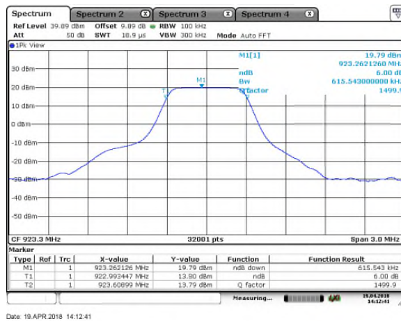
Figure 7.3.2-1: 6dB BW - LCH , SF=7
