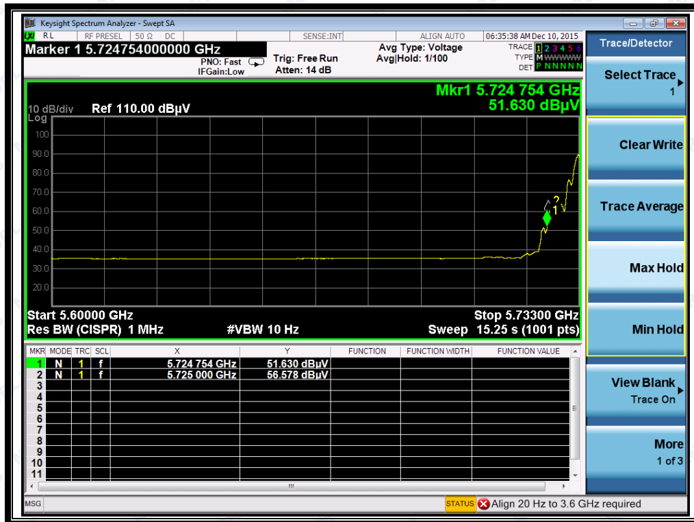
(Plot 1 AV @ Lowest Channel : 5733 MHz)
