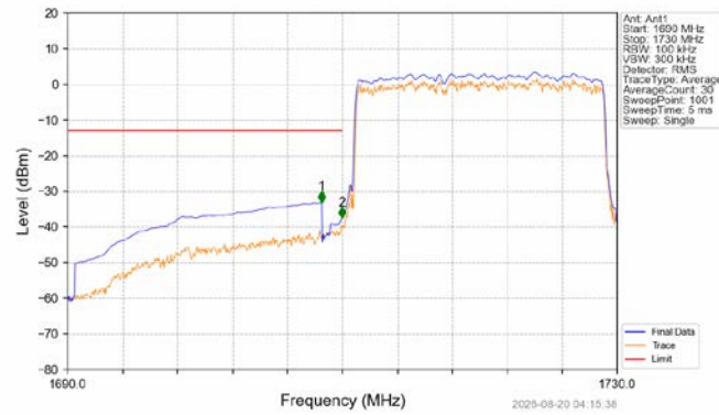
Band4_20MHz_16QAM_LCH_1720MHz_RB_100_0_NTNV
