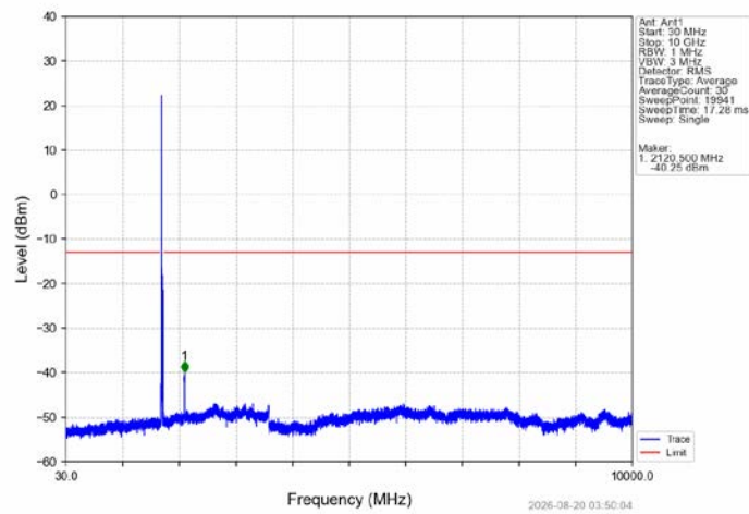
Band4_15MHz_QPSK_LCH_1717.5MHz_RB_1_0_NTNV
