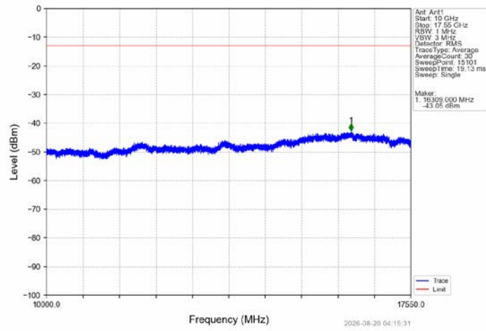
Band4_20MHz_16QAM_LCH_1720MHz_RB_100_0_NTNV
