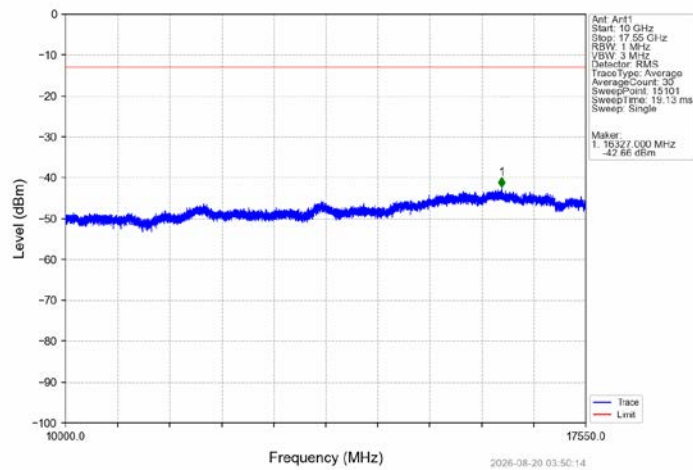
Band4_15MHz_QPSK_LCH_1717.5MHz_RB_1_0_NTNV
