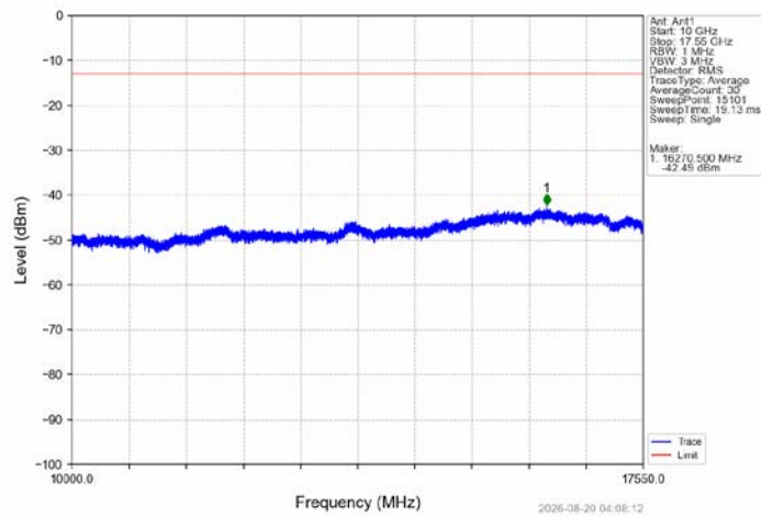
Band4_20MHz_QPSK_LCH_1720MHz_RB_1_0_NTNV
