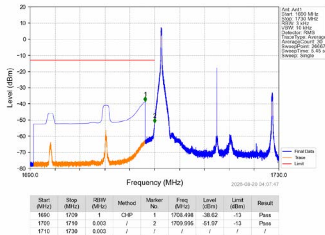
Band4_20MHz_QPSK_LCH_1720MHz_RB_1_0_NTNV
