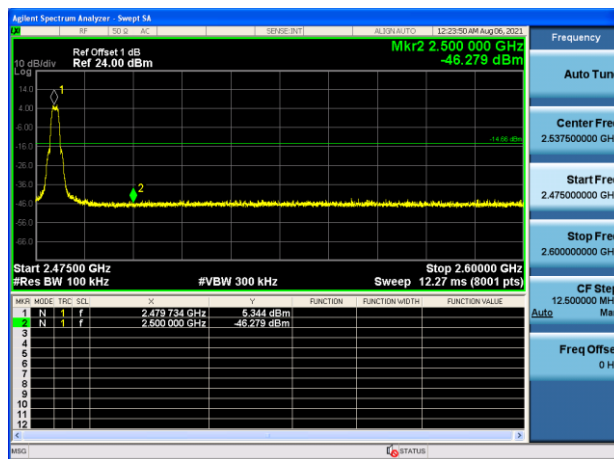
Mode 1 / CH26(2480MHz)
