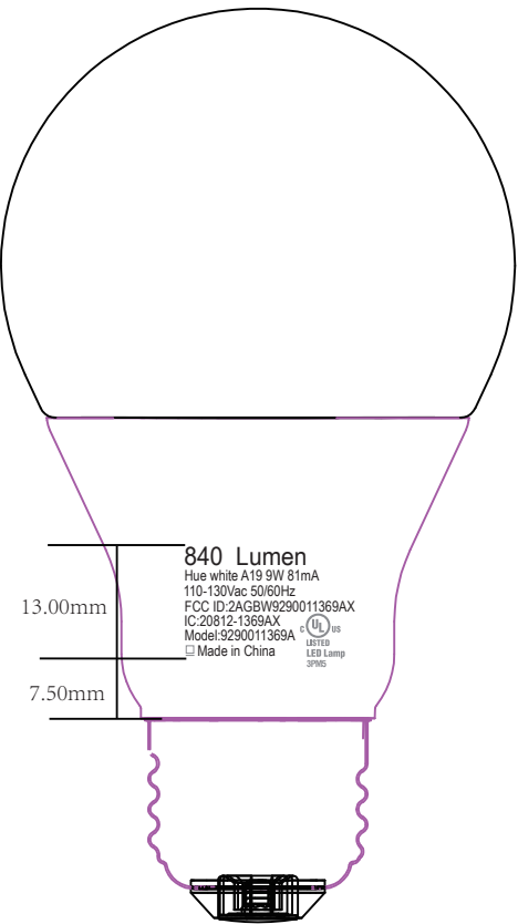
LEFT SIDE
