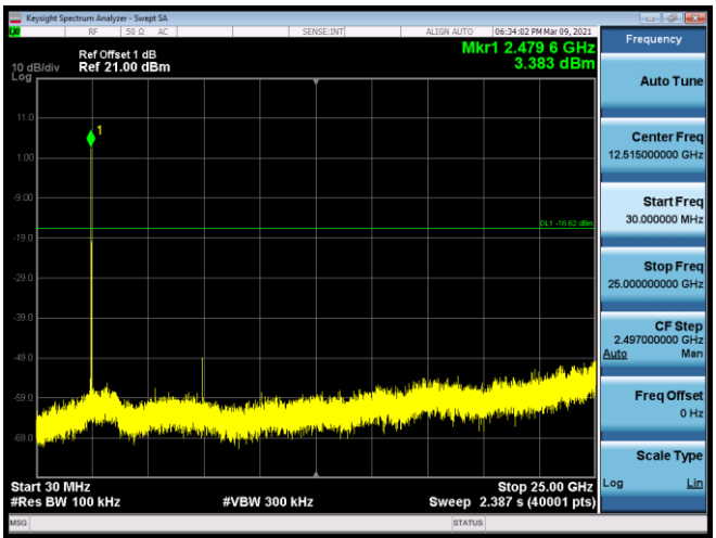
Mode 1 / CH26(2480MHz)
