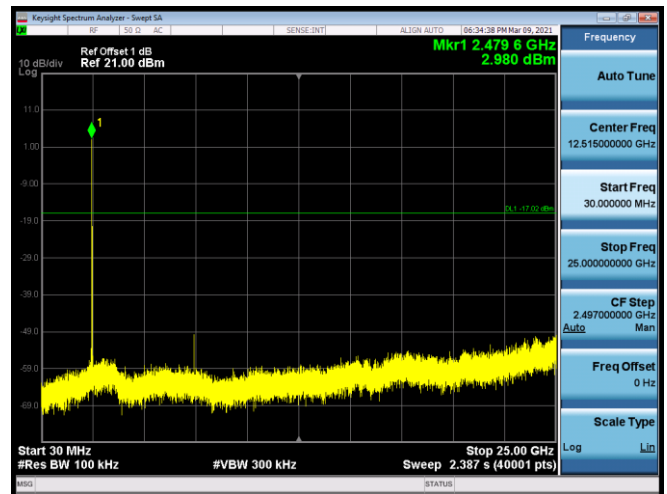
Mode1/CH26/2480MHz
