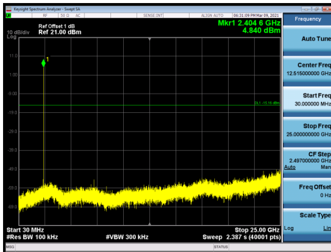
Mode1/CH11/2405MHz
