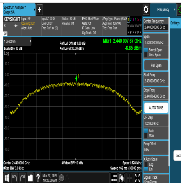
BLE_500K-Ant1-2440-PASS
