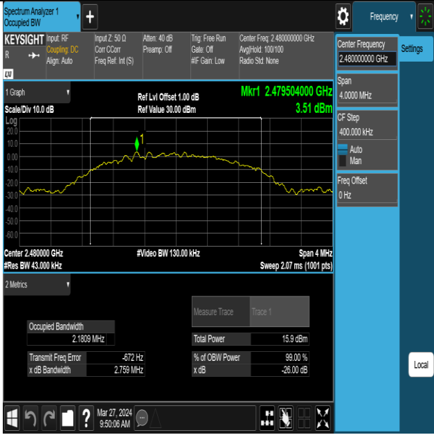
BLE_2M-Ant1-2480
