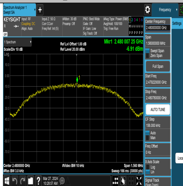
BLE_500K-Ant1-2480-PASS
