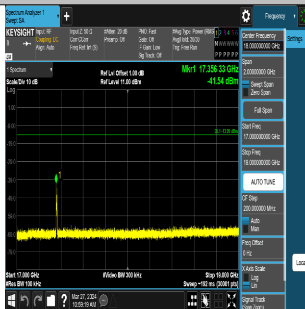
ZIGB-Ant1-2480-17000~19000-PASS
