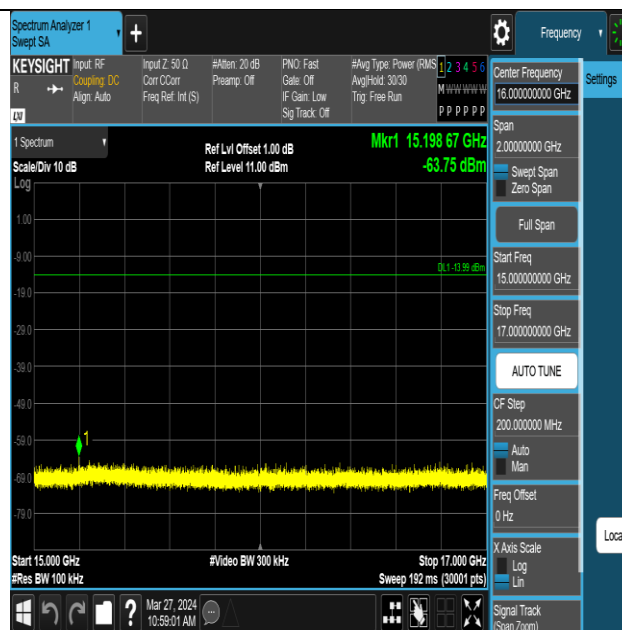
ZIGB-Ant1-2480-15000~17000-PASS
