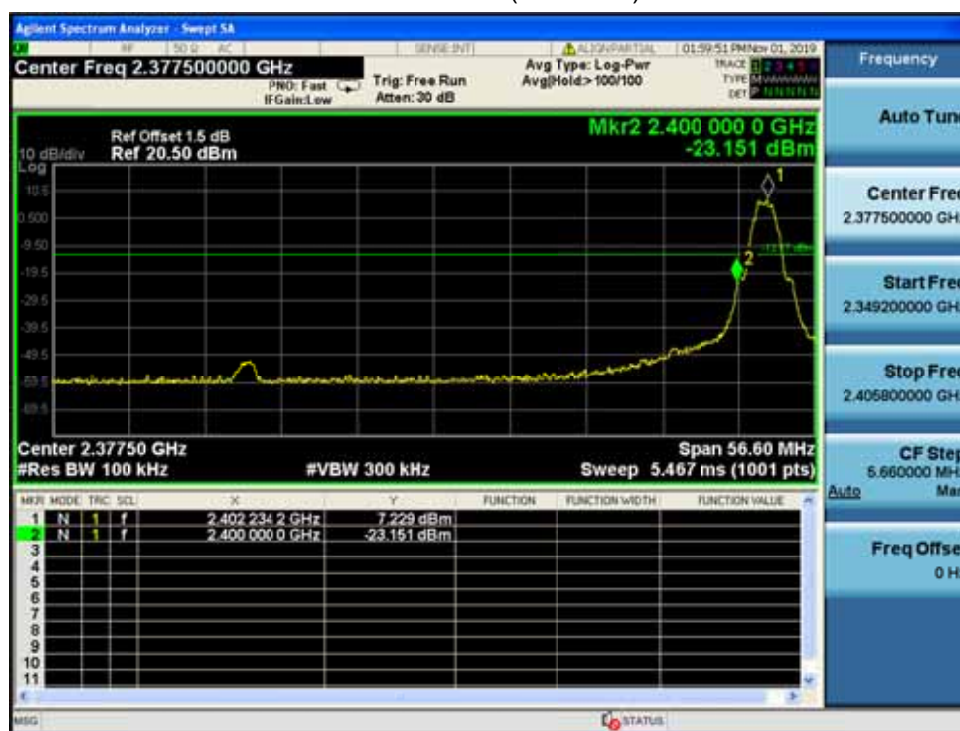
Mode 2 CH00(2402MHz)
