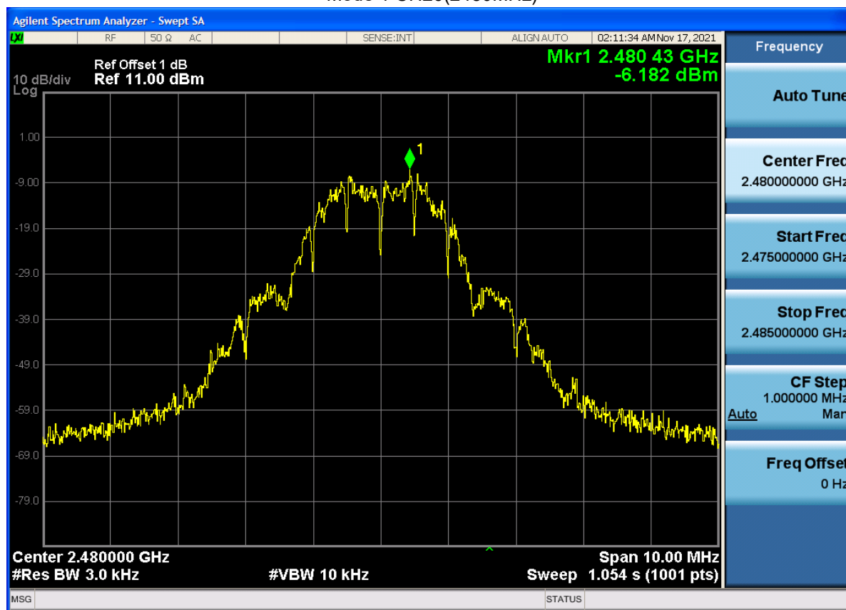
Mode 1 CH26(2480MHz)
