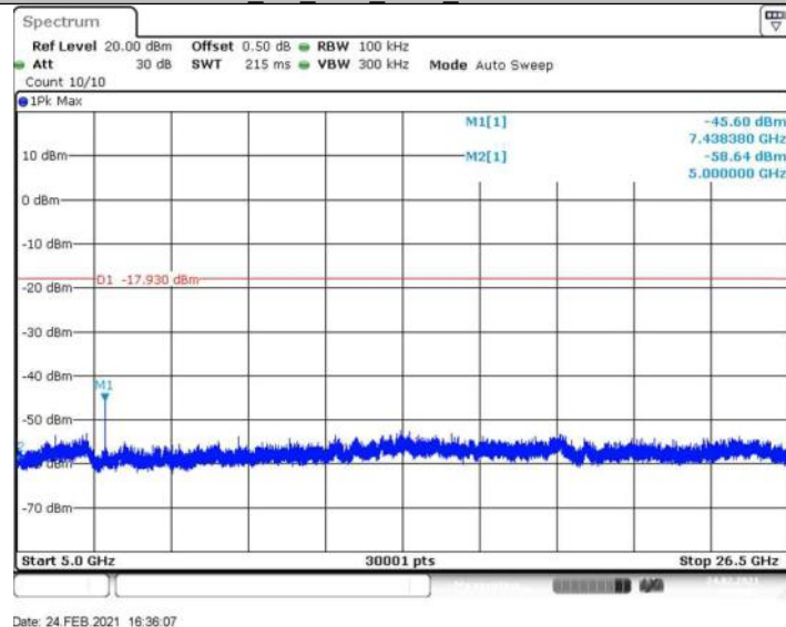
BLE 500K Ant1 2402 0~Reference
