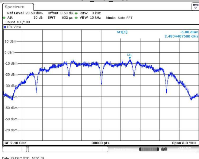
ZIGB_Ant1_2480
