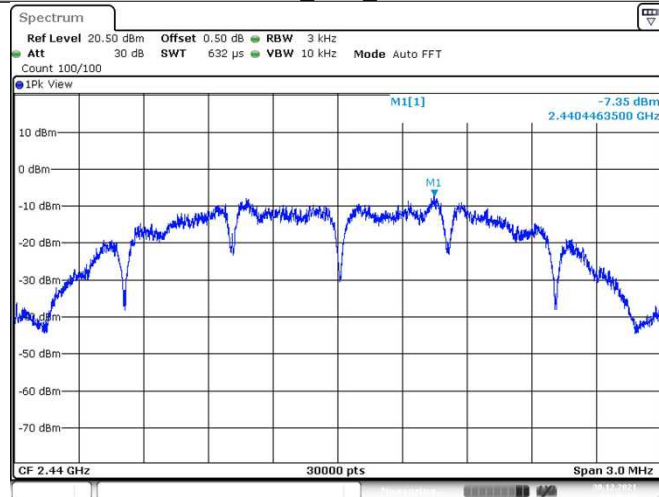
ZIGB_Ant1_2440
