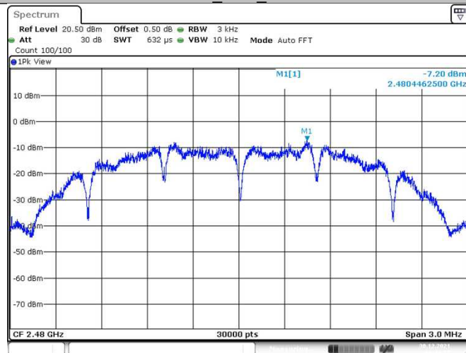
ZIGB_Ant1_2480
