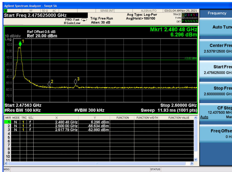
Mode 1 CH26(2480MHz)
