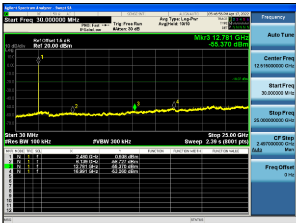
Mode 1 / CH26(2480MHz)
