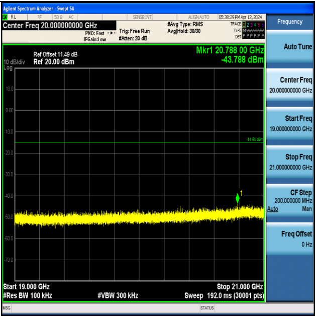
ZIGB-Ant1-2480-19000~21000-PASS
