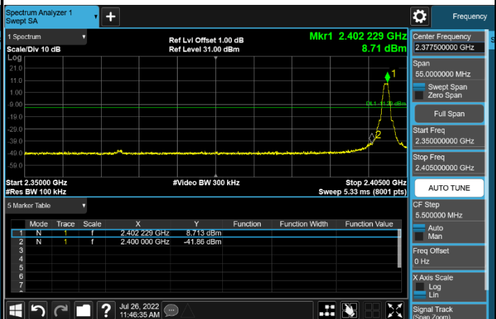
Mode 1 CH00 (2402MHz)
