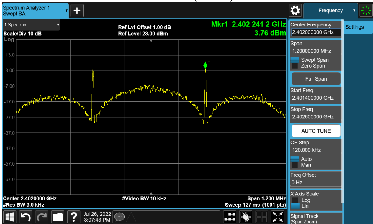
Mode 4 CH00 (2402MHz)
