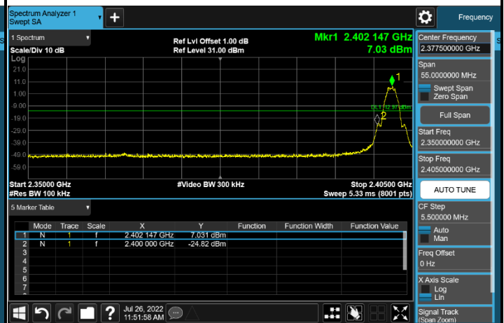
Mode 2 CH00 (2402MHz)
