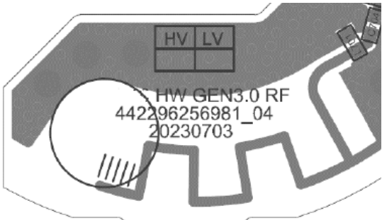
PIFA antenna
