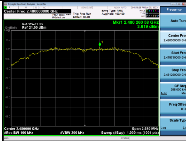
Zigbee_Ant1_2480
