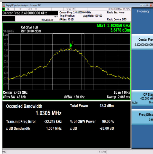
BLE_500K-Ant1-2402
