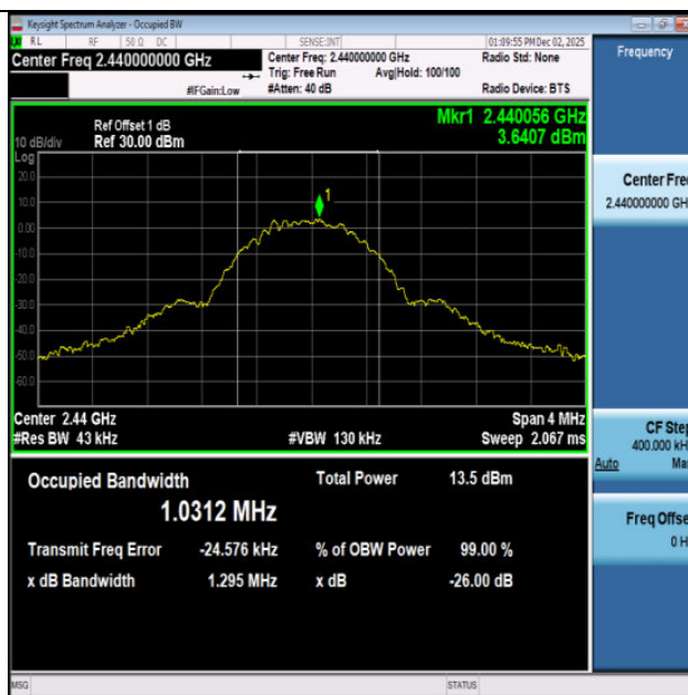
BLE_500K-Ant1-2440
