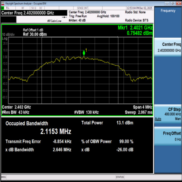
BLE_2M-Ant1-2402
