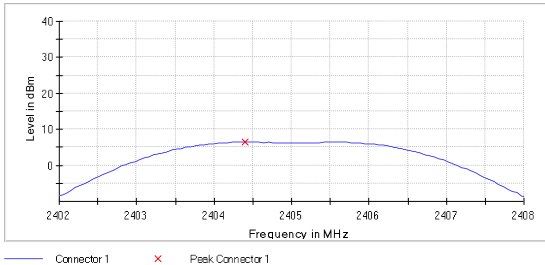
Data of 2405MHz
