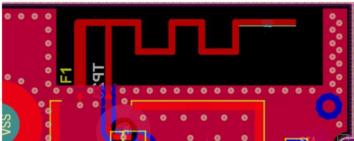
PIFA antenna
