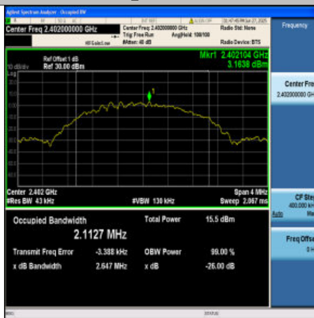
BLE_2M-Ant1-2402
