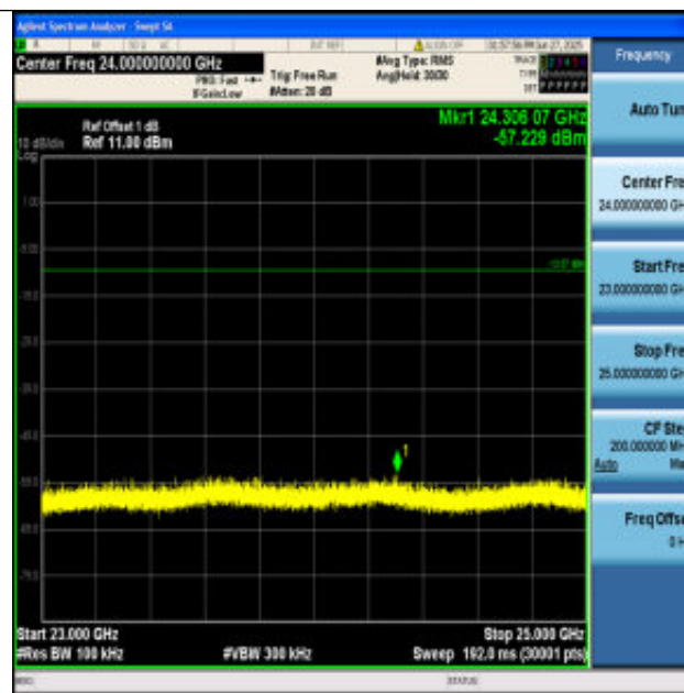
BLE_2M-Ant1-2440-23000~25000-PASS
