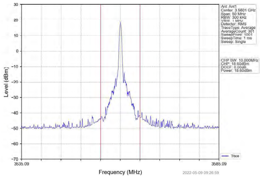
Band48_20MHz_QPSK_LCH_3560MHz_RB_1_50_NTNV
