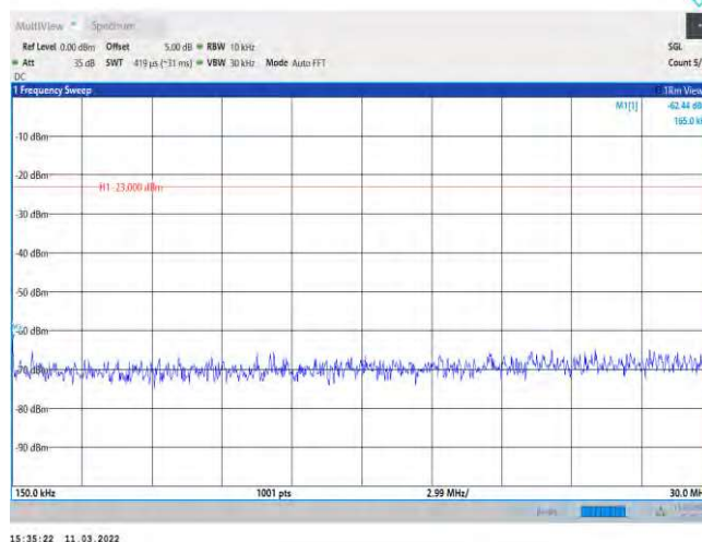
Band71-20MHz-QPSK-133222-1RB#0-Range2:0.15~30MHz
