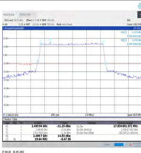
1-N41-30-20-L-3-DFT-16QAM-Outet_Full-50@0-Ant-1-17.935-19.640-≤20-PASS
