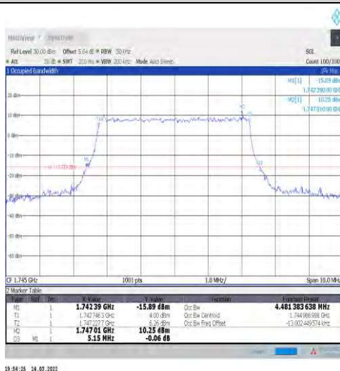
1-N66-15-5-M-6-CP-QPSK-Outer_Full-25@0-Ant1-4. 481-5.150-≤5-PASS
