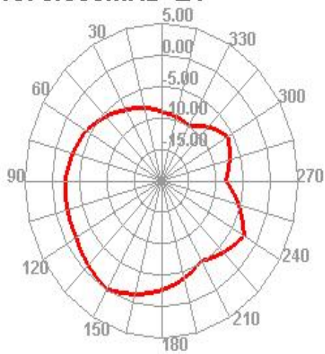
1575.000MHz E1
