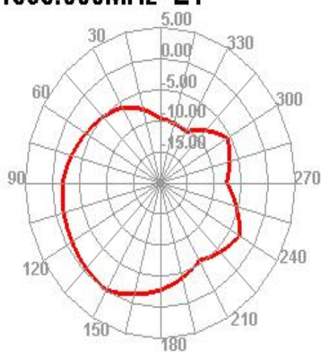
1595.000MHz E1
