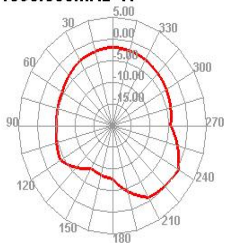
1595.000MHz H
