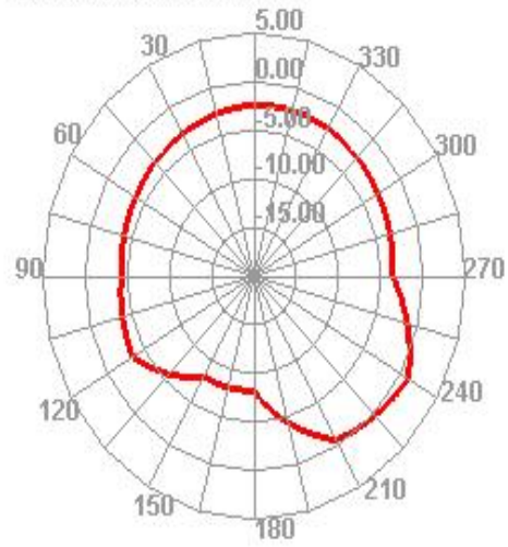
1575.000MHz H
