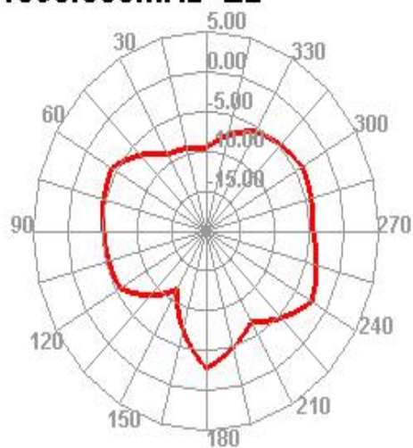
1595.000MHz E2
