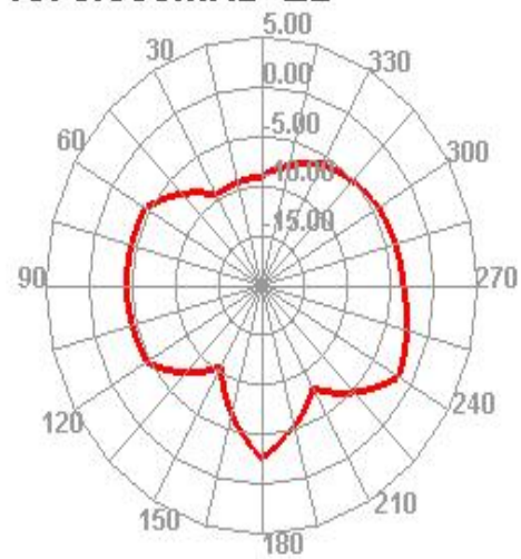
1575.000MHz E2
