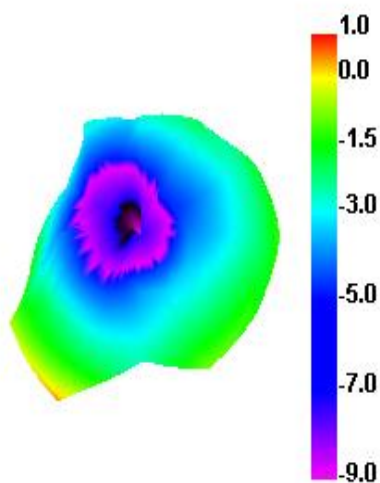
1595.000MHz
